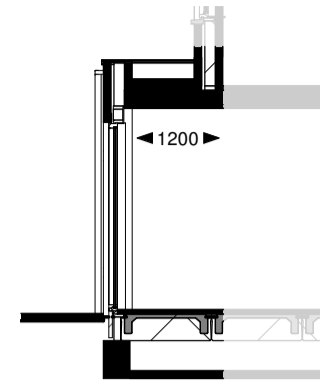
Doorsnede
