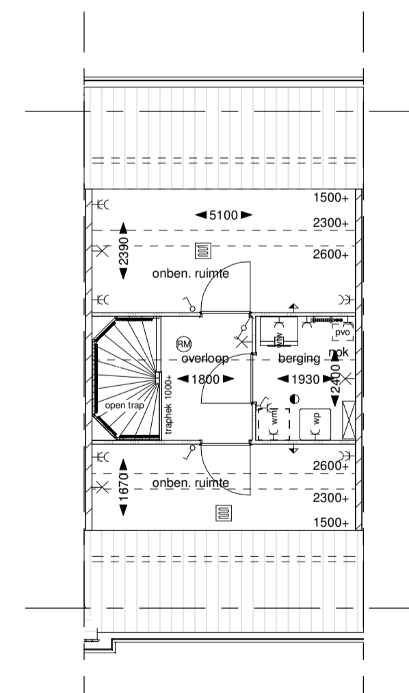
Tweede verdieping
