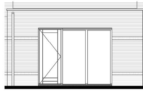
Achtergevel
