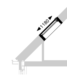
Doorsnede
