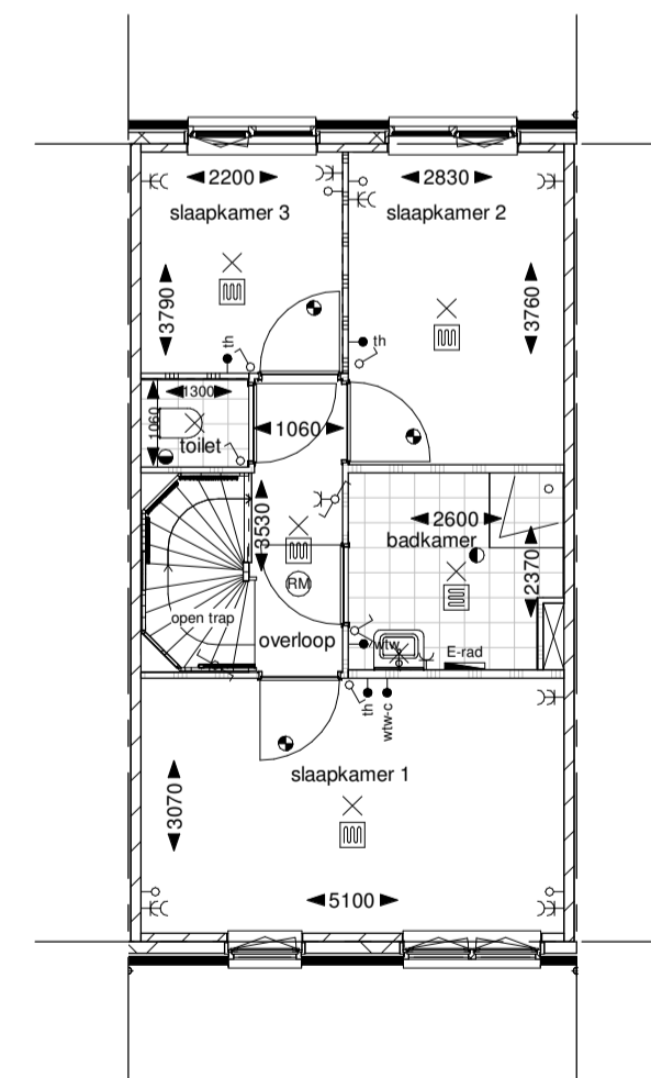
Eerste verdieping
