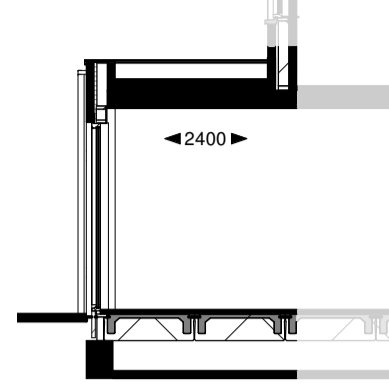
Doorsnede
