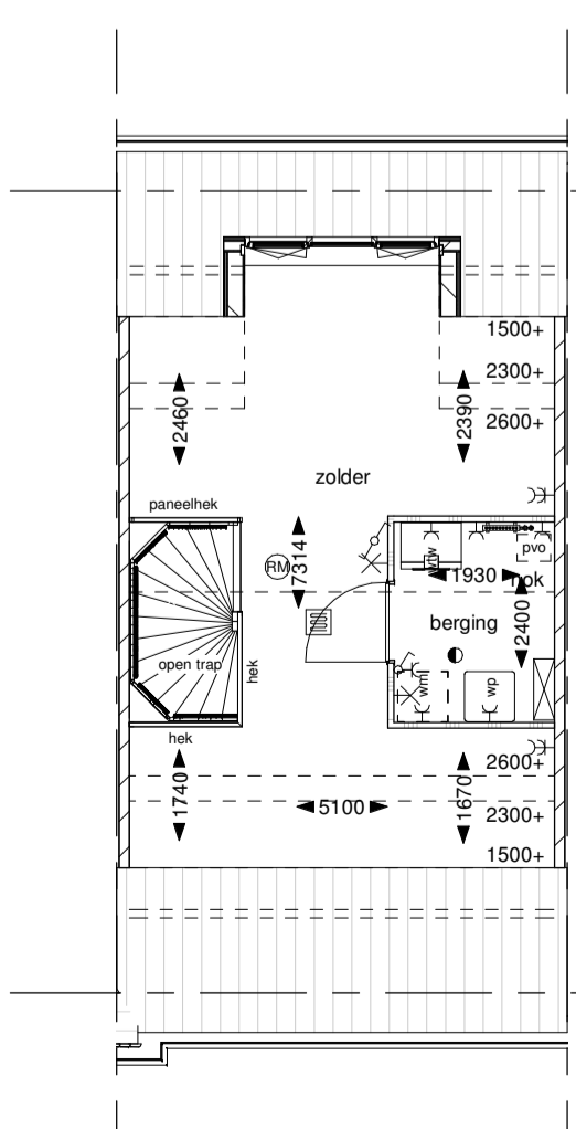
Tweede verdieping
