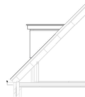
Zijgevel
