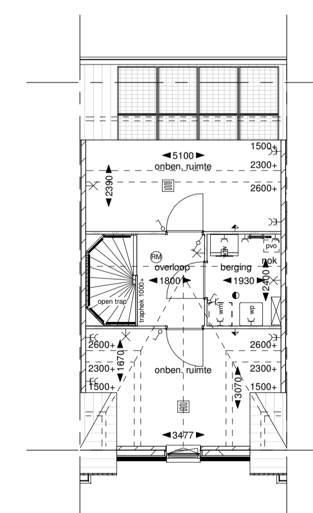
Tweede verdieping
