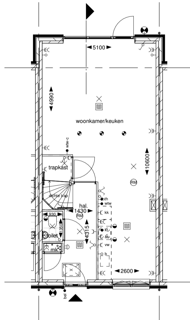
Begane grond
