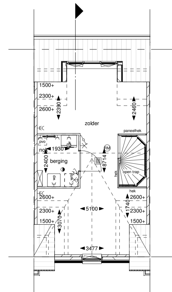
Tweede verdieping
