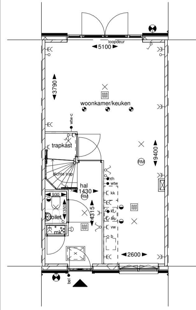
Begane grond
