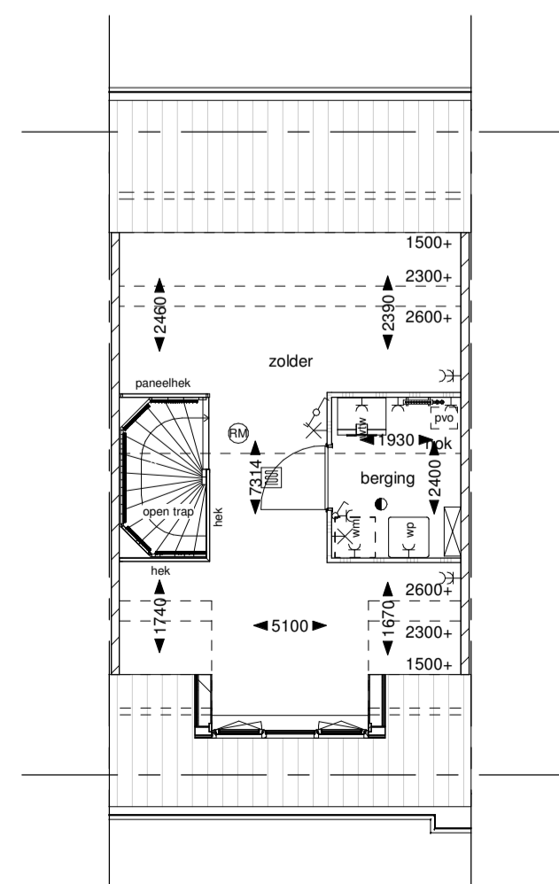
Tweede verdieping
