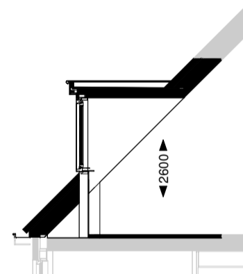
Doorsnede
