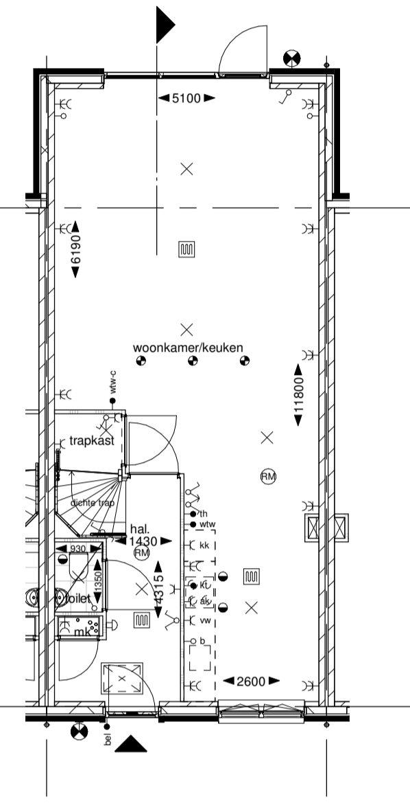
Begane grond
