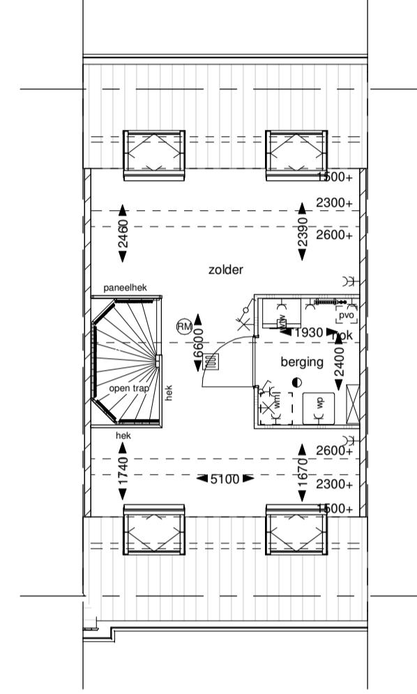
Tweede verdieping
