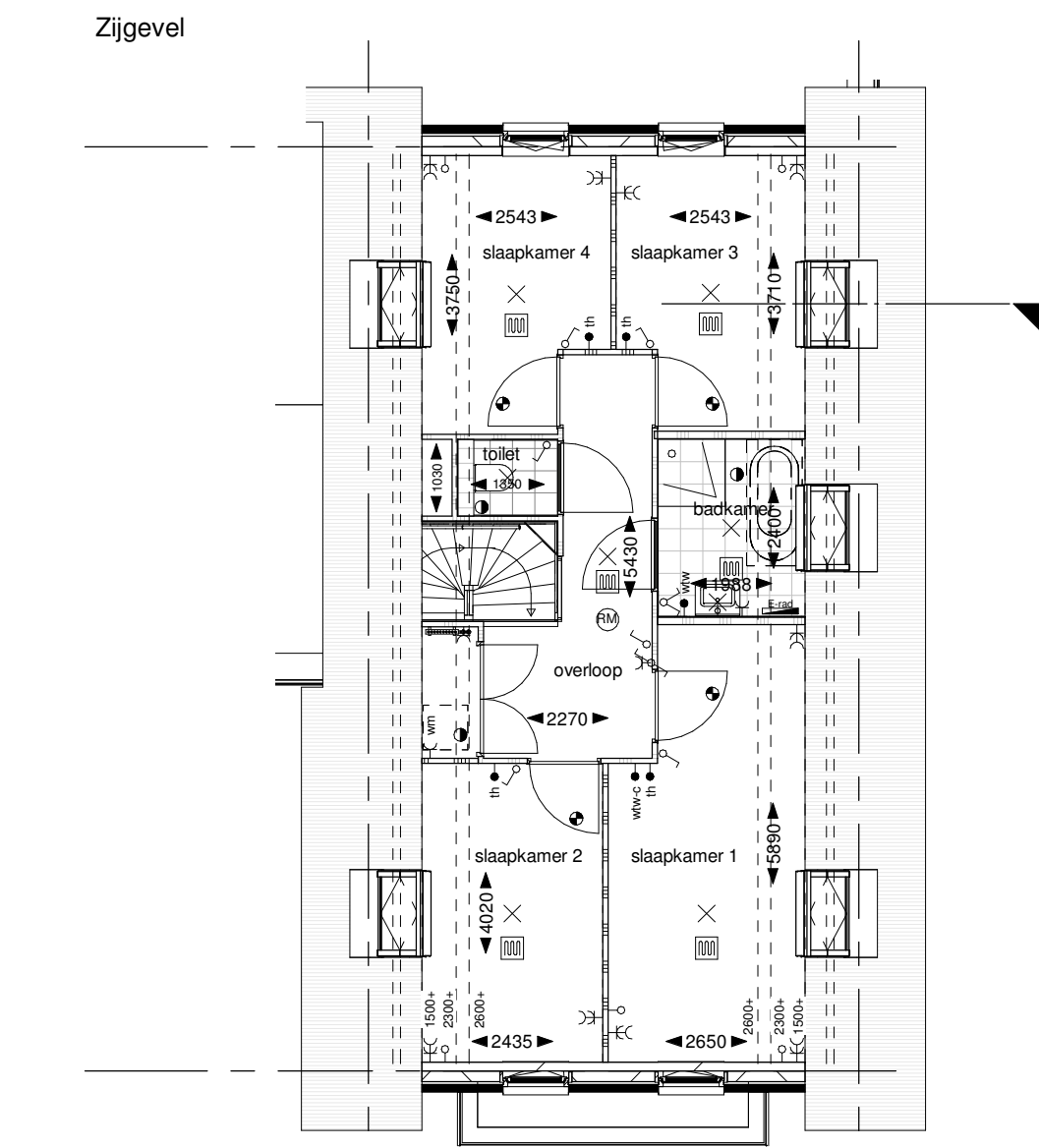
Eerste verdieping
