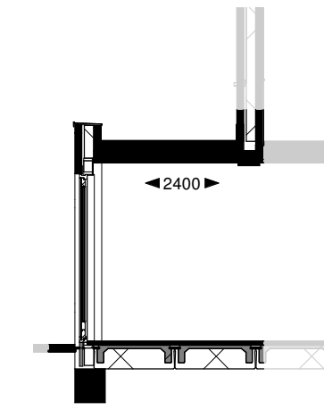
Doorsnede
