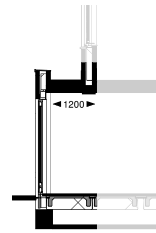
Doorsnede
