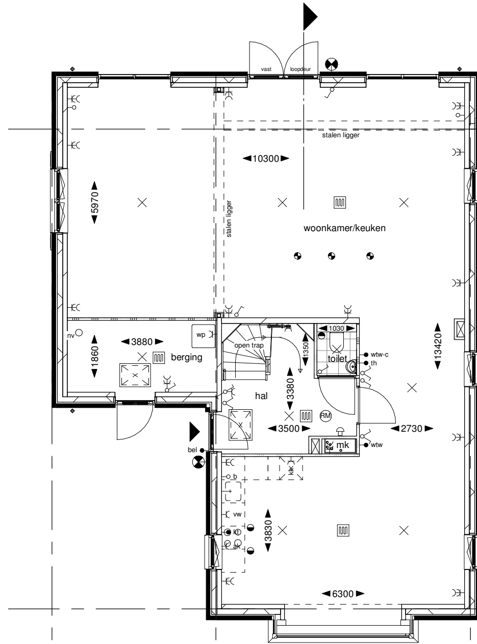
Begane grond
