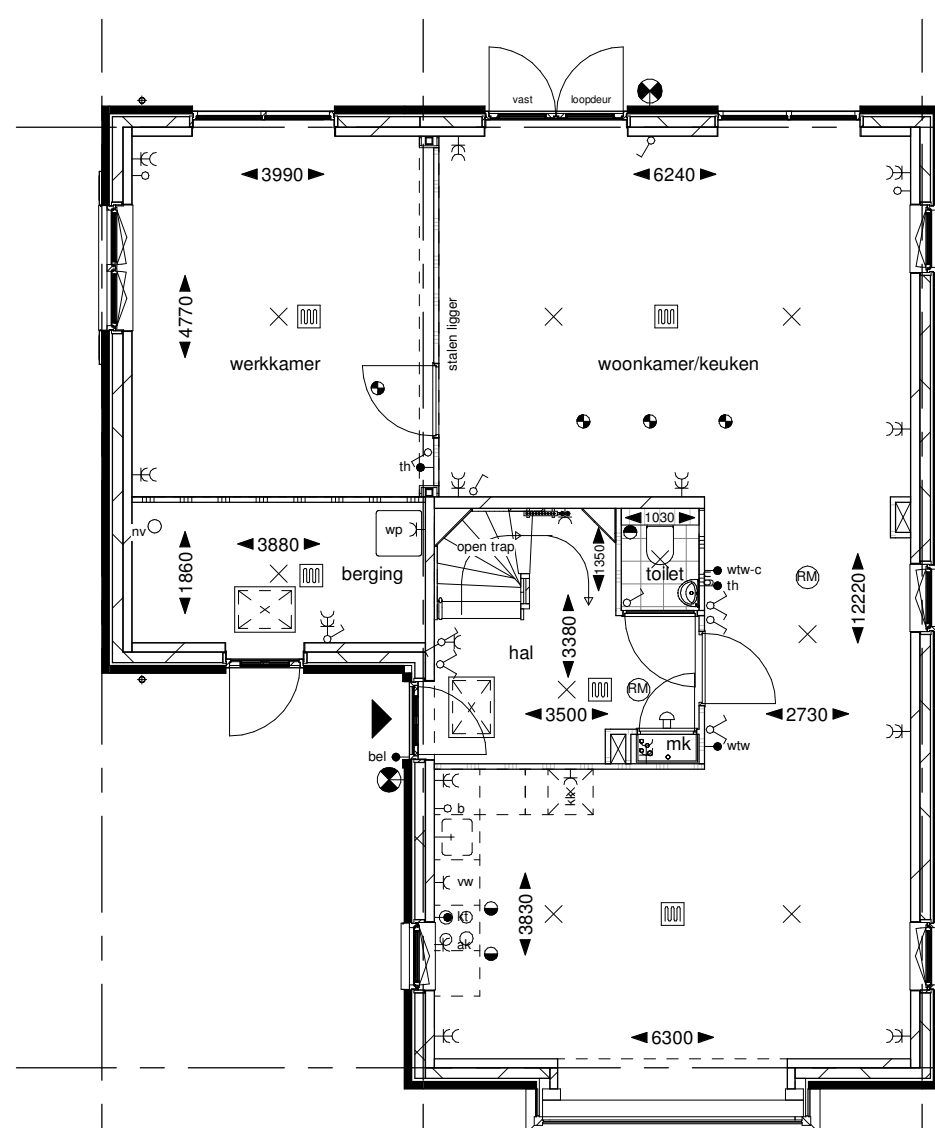
Begane grond
