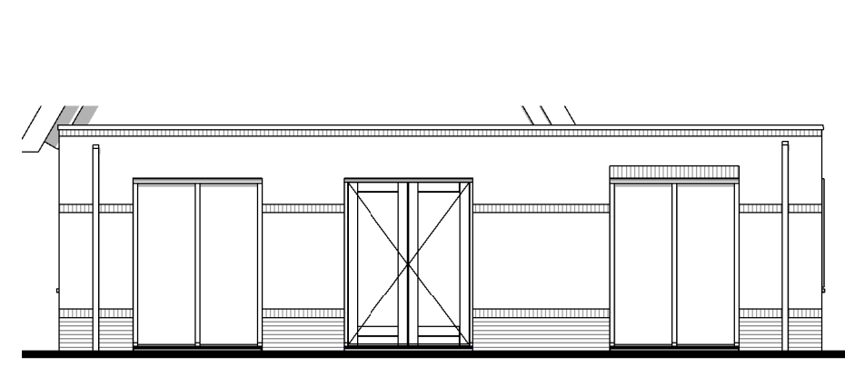
Achtergevel
