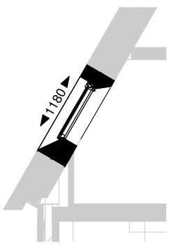
Doorsnede
