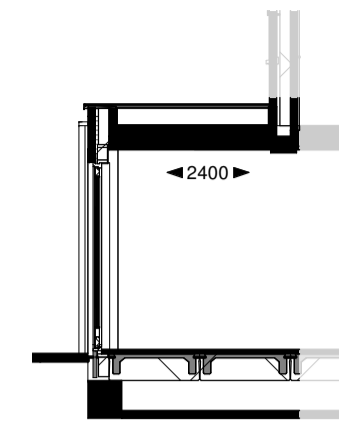
Doorsnede
