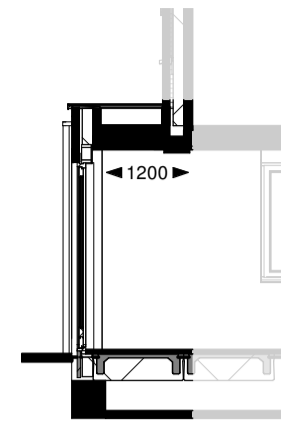
Doorsnede
