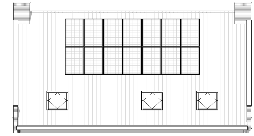
Zijgevel
