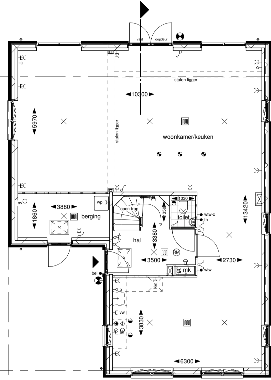
Begane grond
