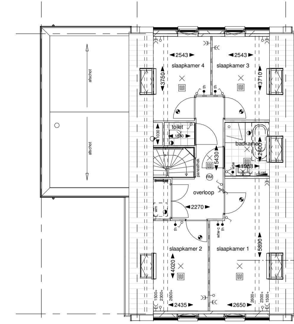
Tweede verdieping
