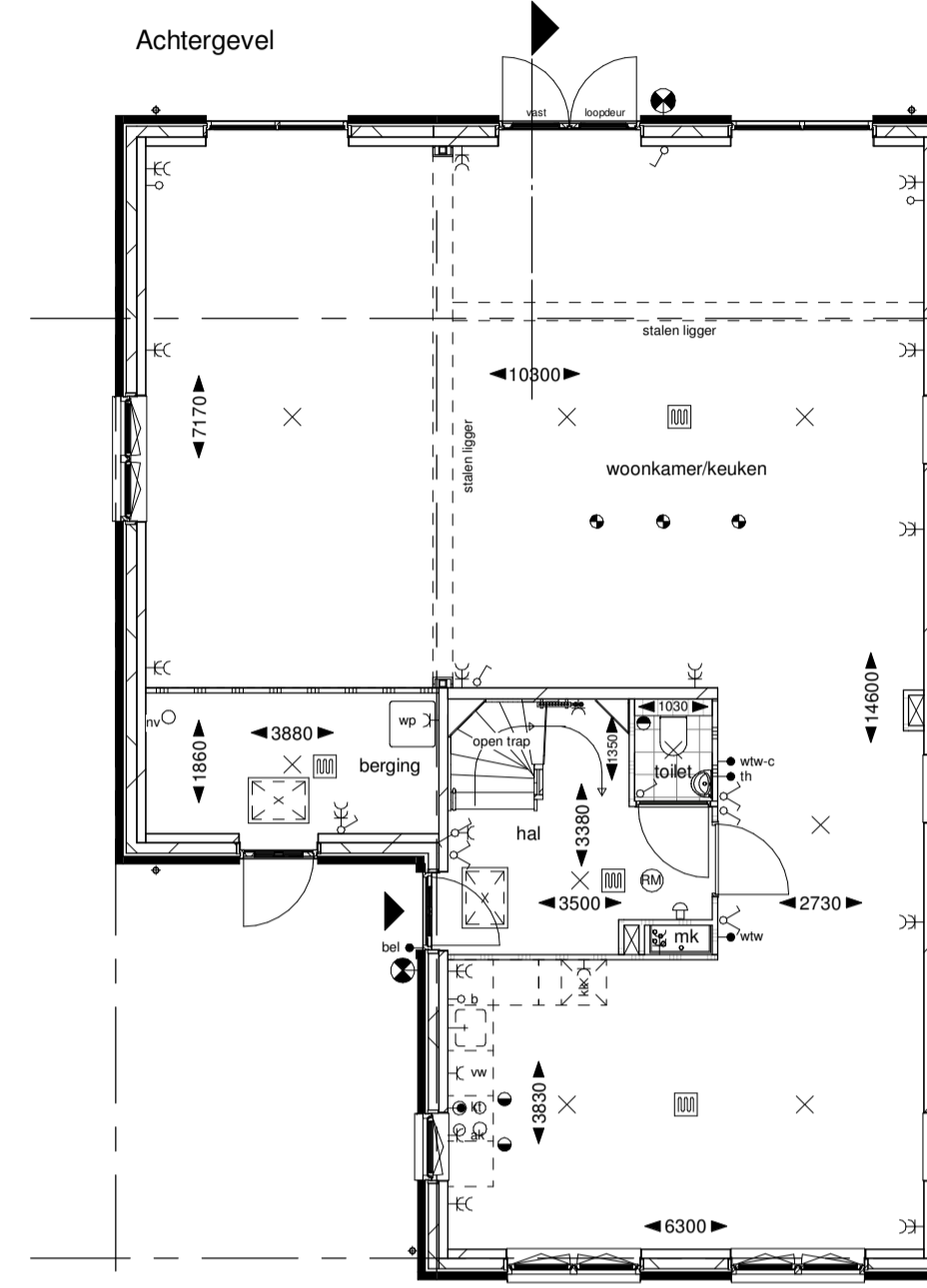
Begane grond
