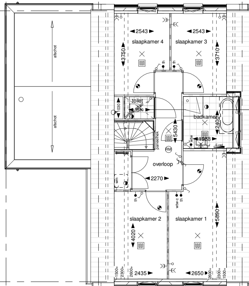
Eerste verdieping
