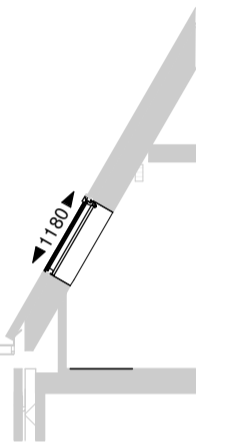
Doorsnede
